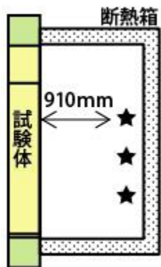
縦断面図
